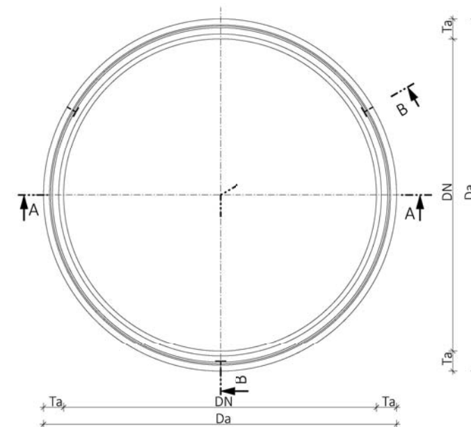
Pohled zdola Skruže DN 2200, DN 2500 a DN 3000
