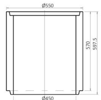
Skruž středová TBV 6D
