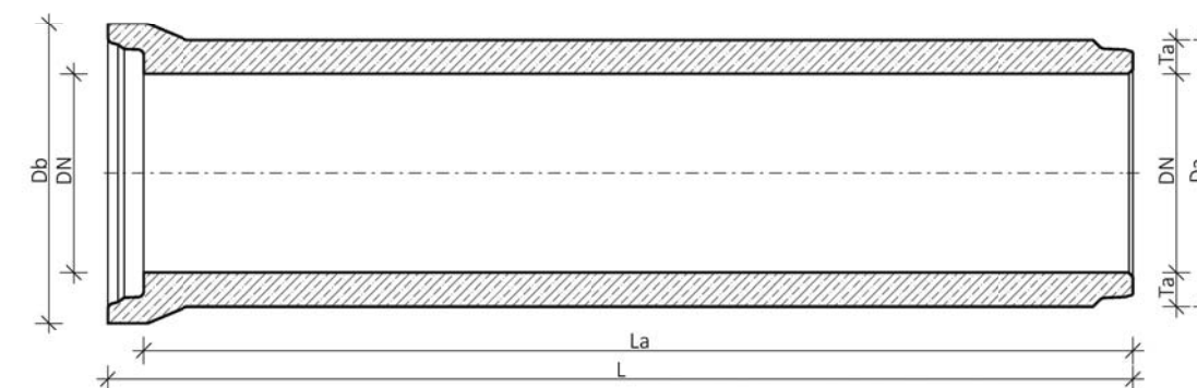
Řez A-A Trouba dříková (TBD / TDD / TZD)
