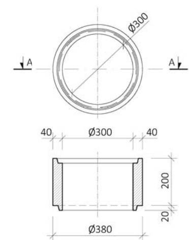
TBD 200b skruže středová
