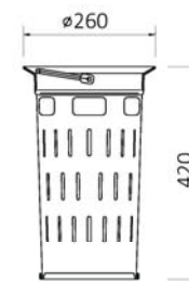
UL kalový koš pozink vysoký
