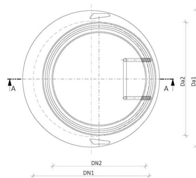
Pohled shora Přejchodové skruže kónické pro DN 1000
