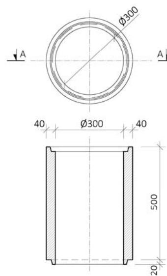
TBD 500b skruže středová
