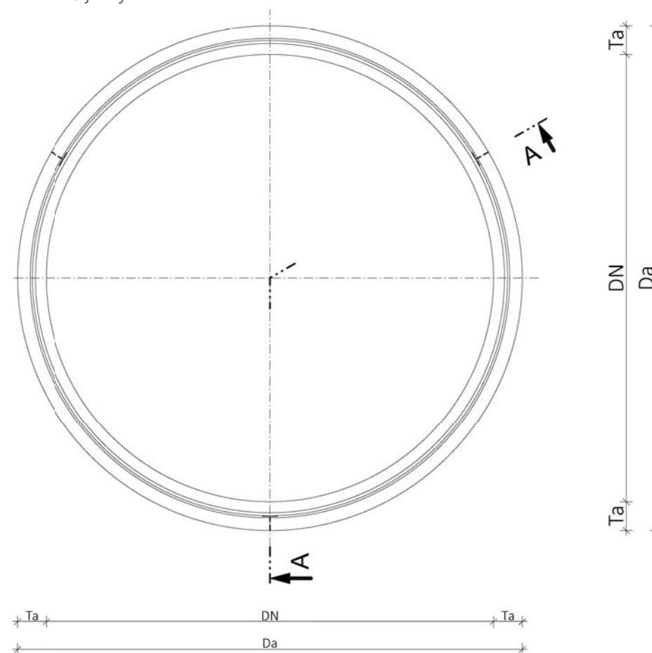
Pohled shora Dno jímky
