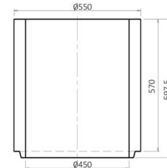
Skruž horní TBV 5D
