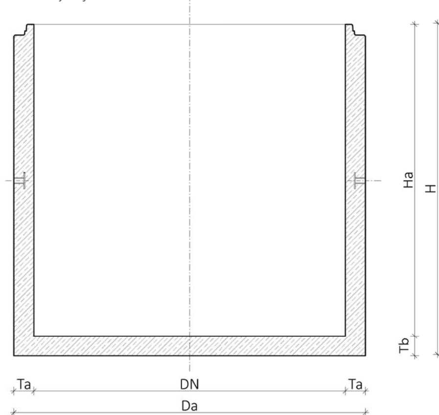
Řez A-A Dno jímky
