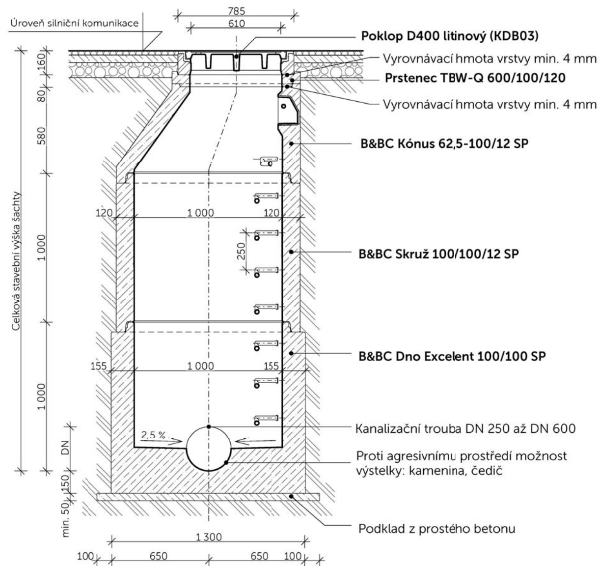
Příklad vstupní šachty DN 1000
