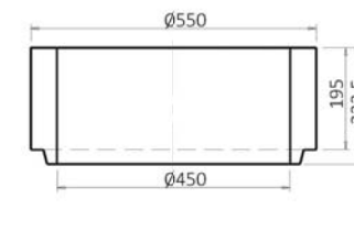
Skruž horní TBV 45C
