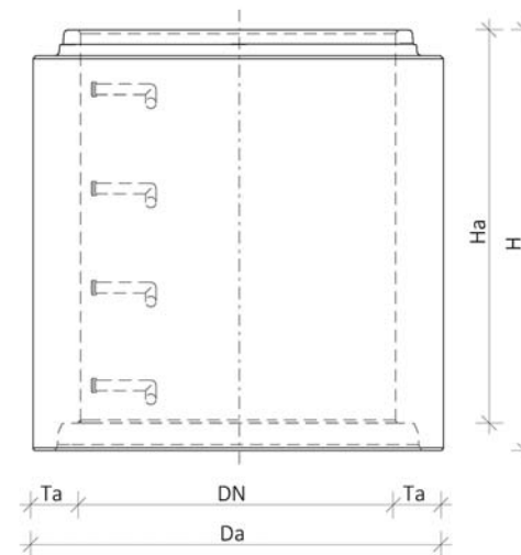
Pohled z boku Skruže DN 800 a DN 1000
