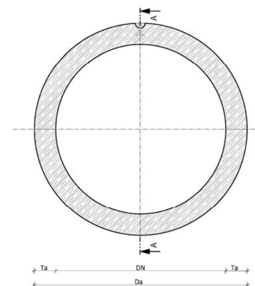
Příčný řez
