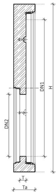
Řez A-A Přechodová stěna dřik
