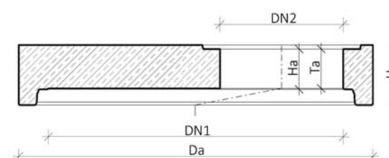
Vizualizace Zákrytové desky pro DN 800 a DN 1700
