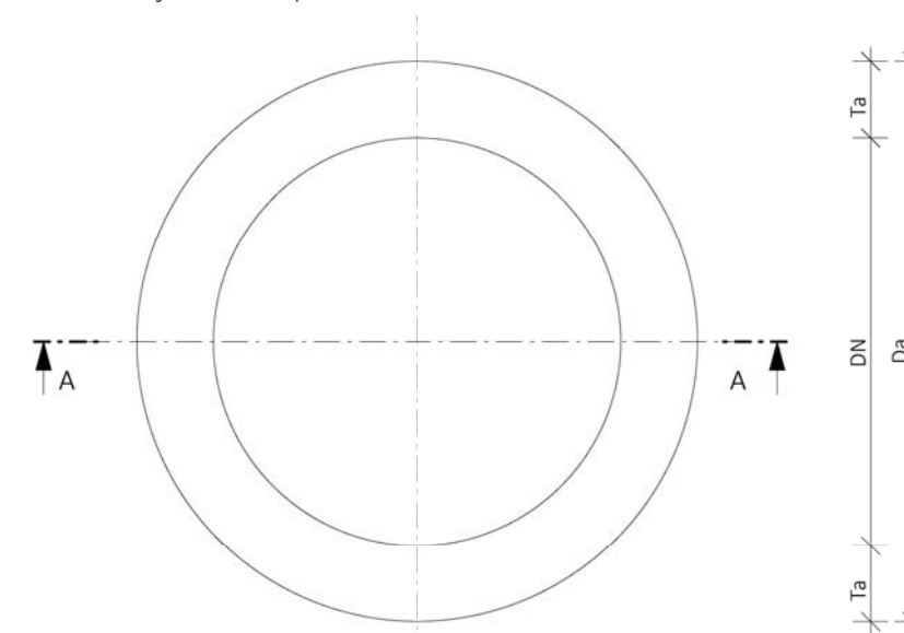
Pohled shora Vyrovnávací prstence DN 800
