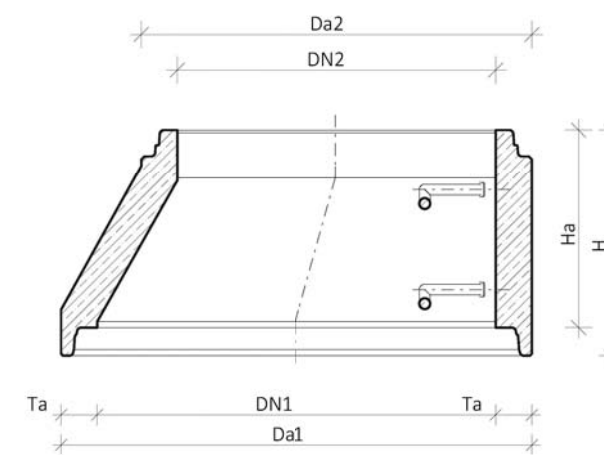
Řez A-A Přejchodové skruže kónické pro DN 1000
