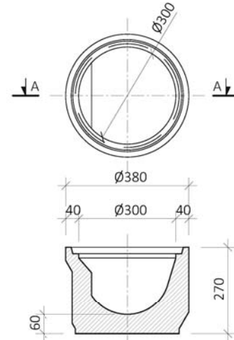
TBD 270 dno s kalovou prohlubní
