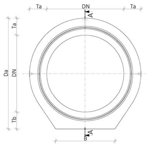
Pohled na dřík Trouba přímá patková (TZPP)
