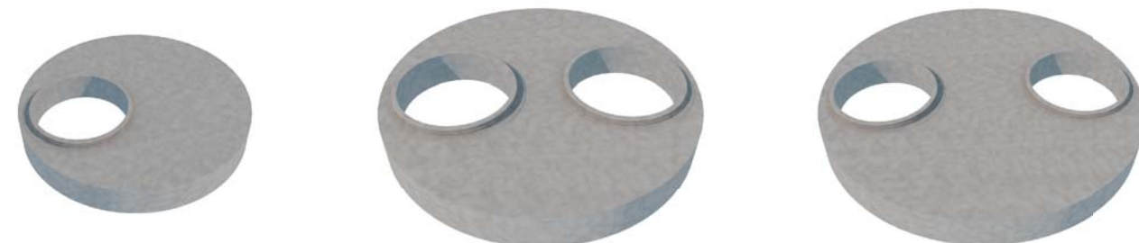
Vizualizace Přečtové desky pro DN 2200 až DN 3000
