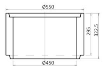
Skruž středová TBV 46A
