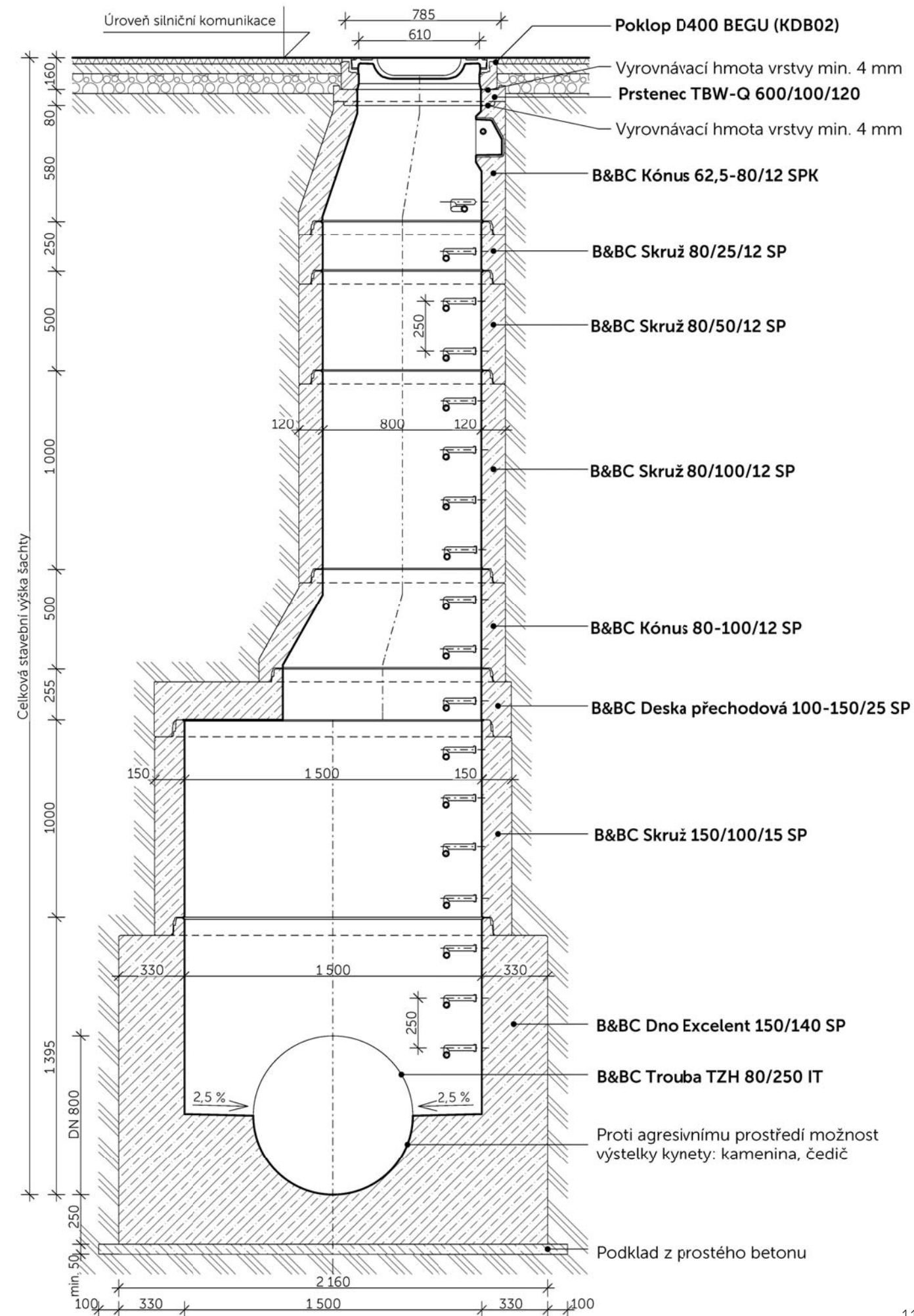
Příklad vstupní šachty DN 1500
