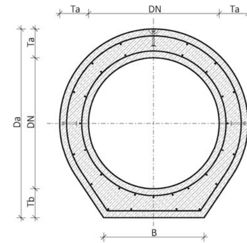
Řez B-B Trouba přímá patková (TZPP)
