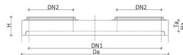
Pohled z boku Přečtové desky pro DN 2200 až DN 3000
