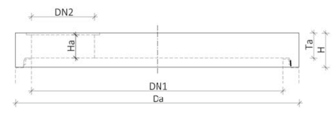
Řez A-A Zákrytové desky pro DN 2200 až DN 3000
