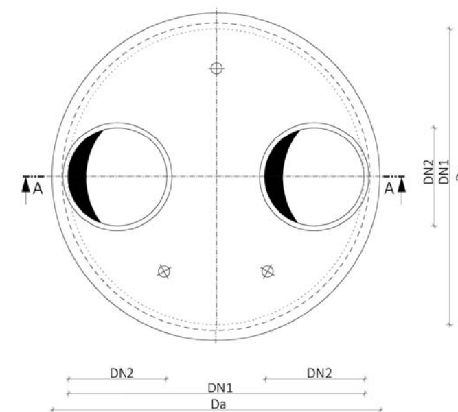
Pohled shora Přečtové desky pro DN 2200 až DN 3000
