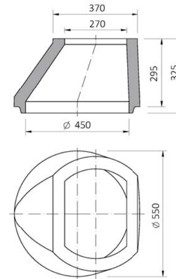
Kónus K11A
