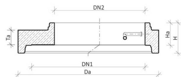
Řez A-A Přečtové desky pro DN 1000 až DN 1700
