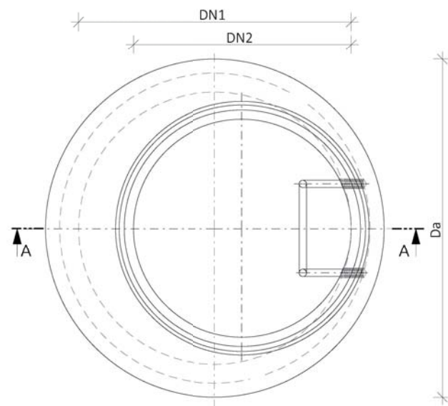
Pohled shora Přečtové desky pro DN 1000 až DN 1700
