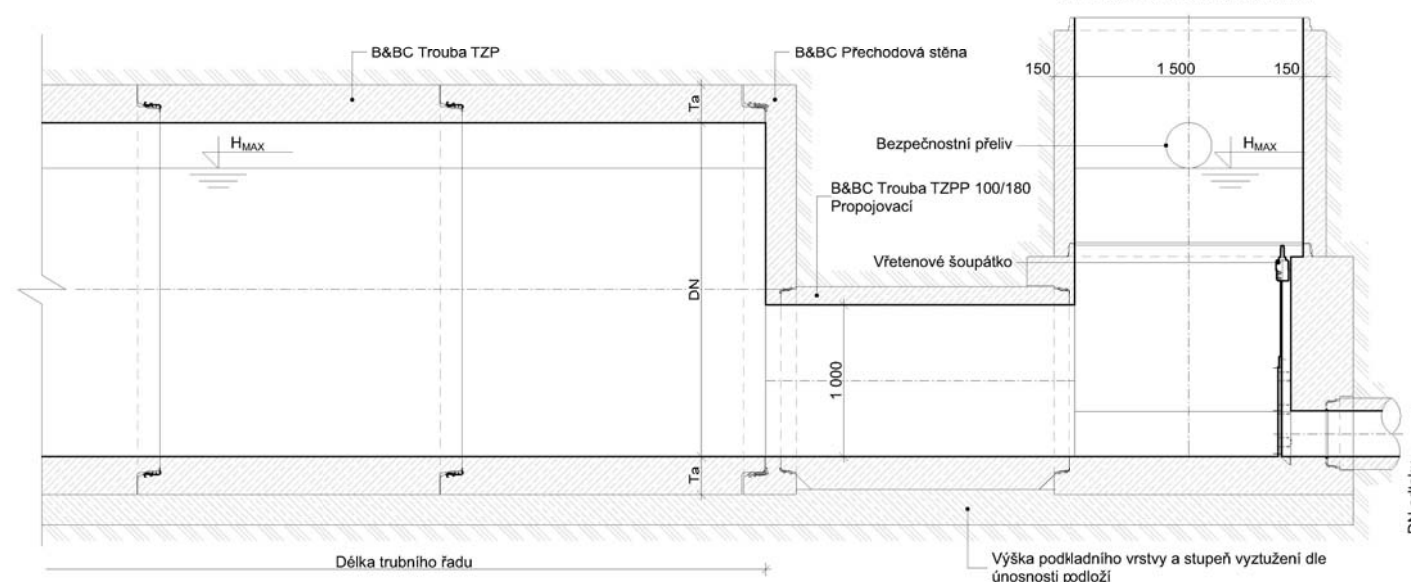
Retence - Odtok
