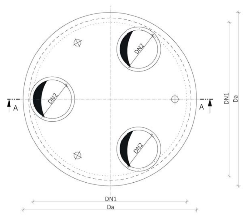
Pohled shora Zákrytové desky pro DN 2200 až DN 3000
