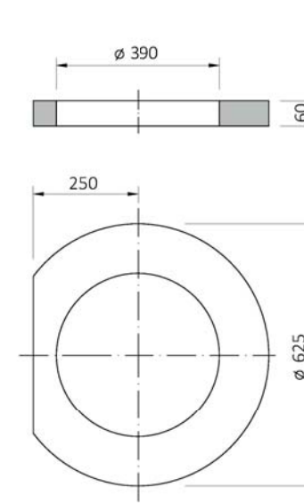
Prstenec vyrovnávací 10A
