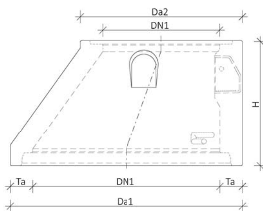
Pohled z boku Zákrytové skruže kónické, tl. stěny 120 mm
