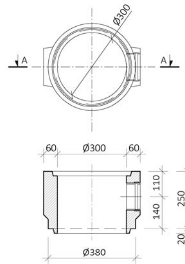
TBD 250 1e skruže s otvorem, 1x DN 100 PVC
