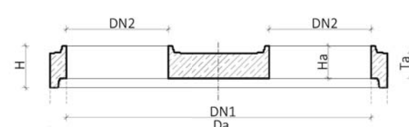
Vizualizace Přečtové desky pro DN 2200 až DN 3000
