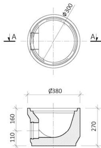
TBD 270a dno s výtokem DN 100 PVC
