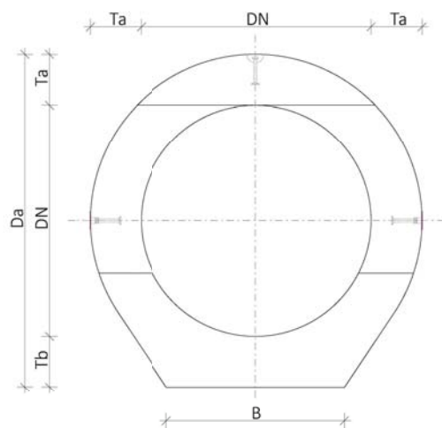
Pohled na vtok Trouba přímá patková vtoková (TZPP)
