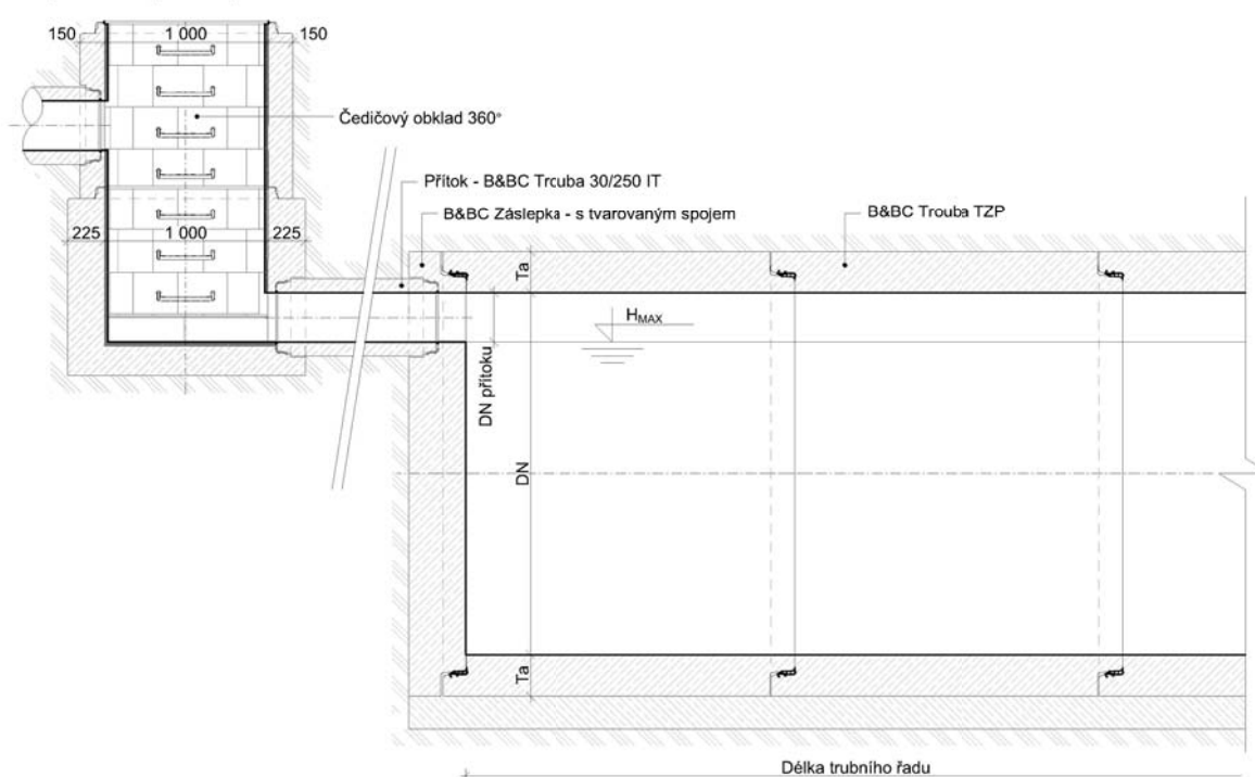
Retence - přítok
