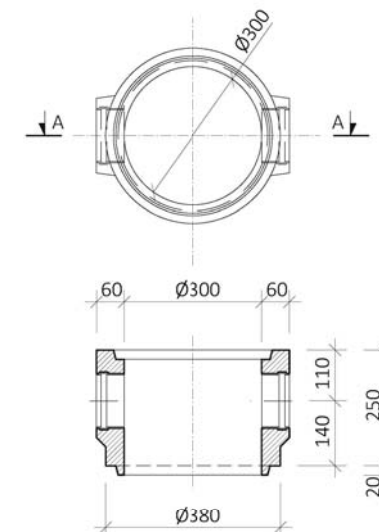
TBD 250 2e skruže s otvorem, 2x DN 100 PVC
