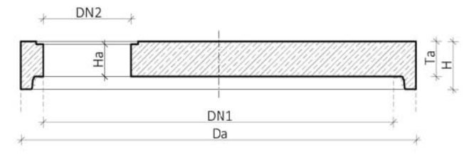
Pohled z boku Zákrytové desky pro DN 2200 až DN 3000
