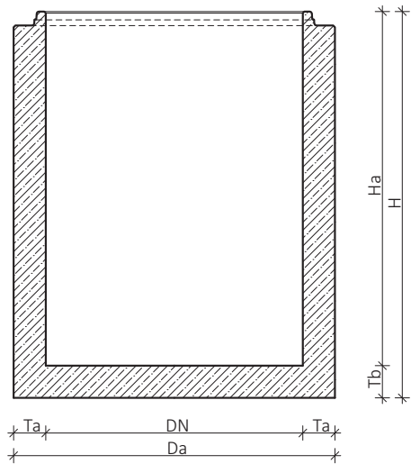
Řez A-A Dno jímky
