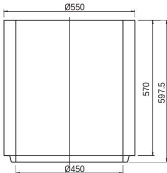
Skruž horní TBV 5D
