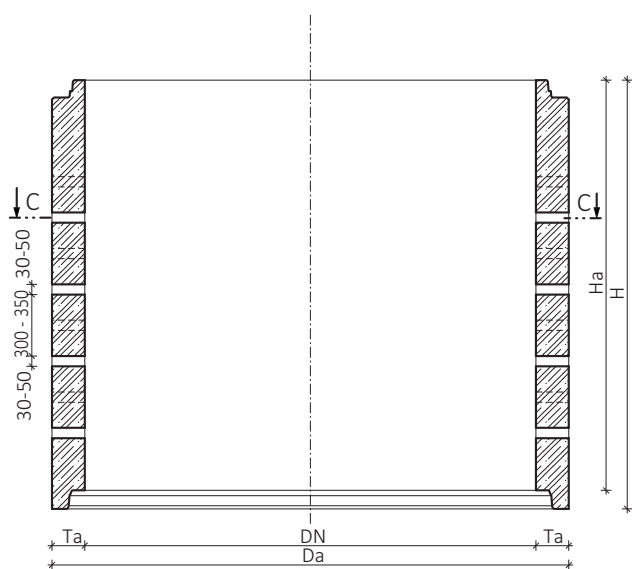
Řez A-A
