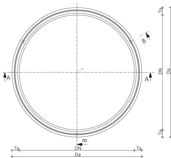
Pohled zdola Skrůže DN 2200, DN 2500 a DN 3000
