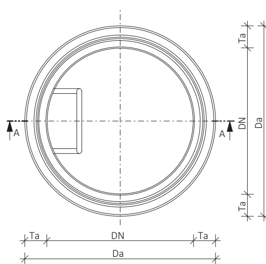
Pohled zdola Skruze DN 800 a DN 1000
