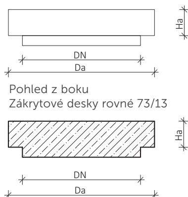
Řez A-A Zákrytové desky rovné 73/13
