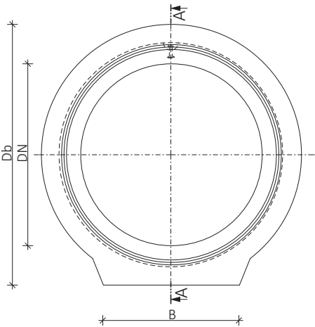
Pohled na hrdlo Trouba hrdlová patková (TBHP / TZHP)
