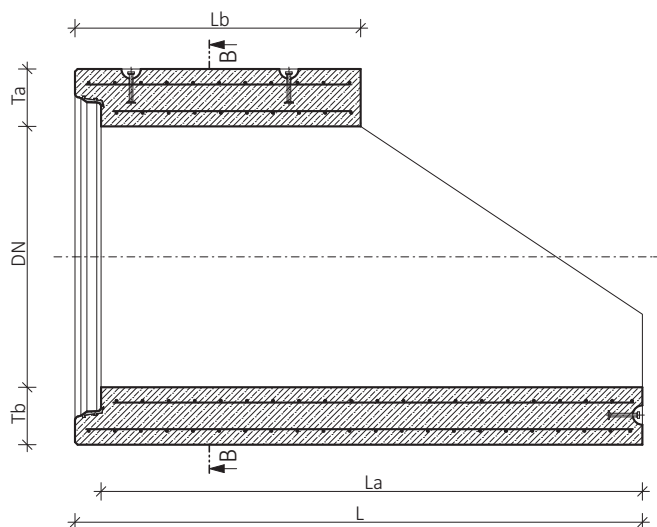
Řez A-A
