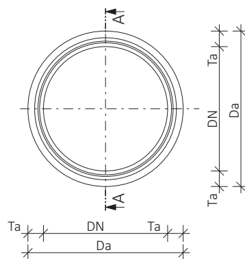
Pohled na dřík Trouba přímá (TBP)
