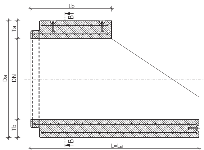
Řez A-A
