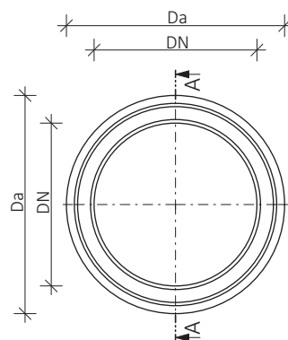
Pohled na dřívko Trouba dřívková (TBD / TDD / TZD)
