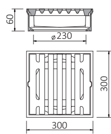
Vtoková mříž KMB125 (B125)
