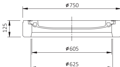
Poklop B125 BEGU bez odvětrání (KBB01)
