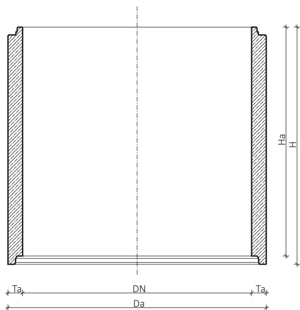
Řez A-A Skrůže DN 2200, DN 2500 a DN 3000
