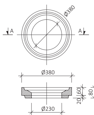
TBD držák kalového koše
