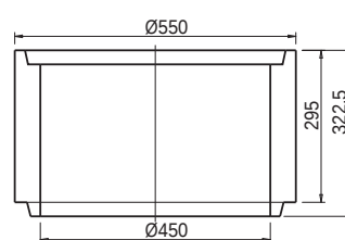
Skruž středová TBV 46A
