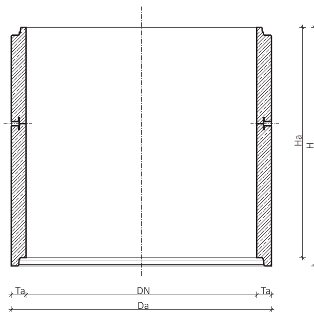
Řez B-B Skrůže DN 2200, DN 2500 a DN 3000
