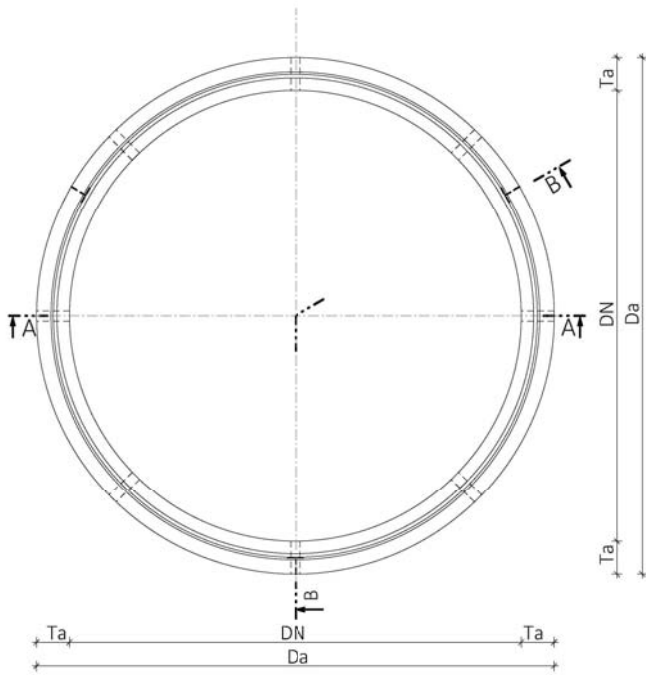
Pohled shora Skruze perforované DN 2200 až DN 3000
