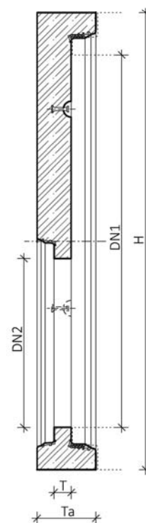
Řez A-A Přechodová stěna dřív
