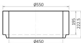
Skruž horní TBV 45C
