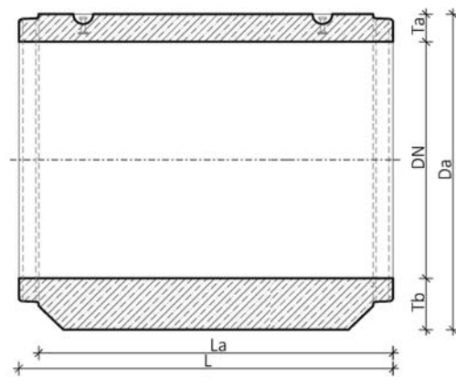
Řez A-A Trouba dřívková patková (TBDP / TZDP)
