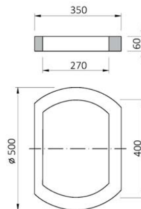
Prstenec vyrovnávací 10B
