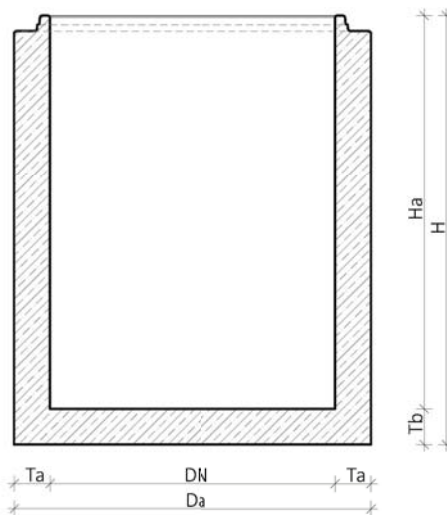
Řez A-A Dno jímky
