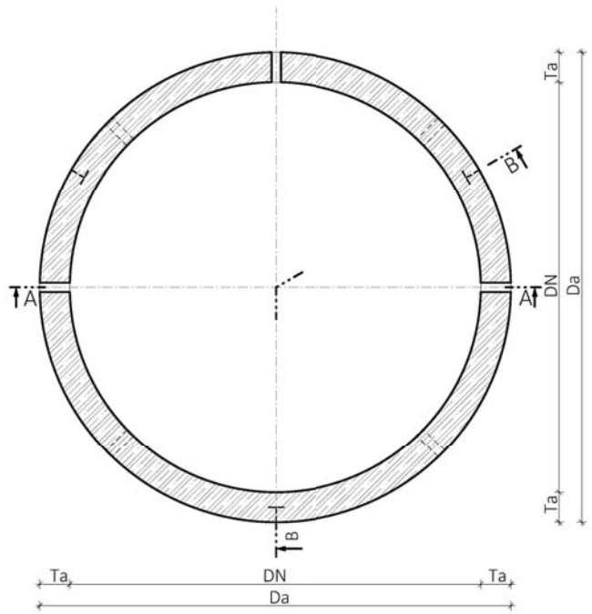
Řez C-C Skruze perforované DN 2200 až DN 3000
