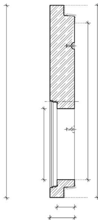
Řez A-A Přechodová stěna hrdlo
