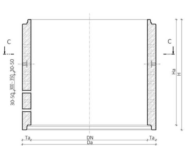
Řez B-B Skruze perforované DN 2200 až DN 3000
