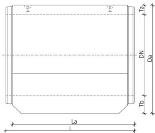
Pohled z boku Trouba dřívková patková (TBDP / TZDP)
