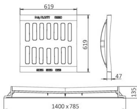
Mříž plastová s litinovým rámem C250 na horskou vpust
