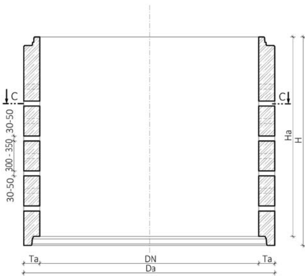
Řez A-A Skruze perforované DN 2200 až DN 3000
