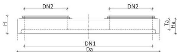
Pohled z boku Přejchodové desky pro DN 2200 až DN 3000
