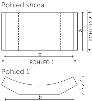
B&BC Žlab 33-60
