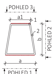
Pohled shora
