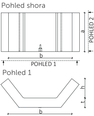
B&BC Žlab 33-60
