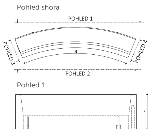
Pohled 2
