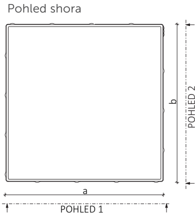
B&BC Obdélník 40-20-6
