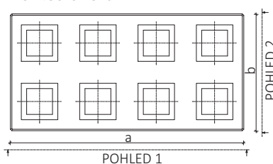
Pohled shora
