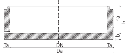
Řez A-A
