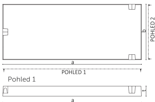
Pohled shora
