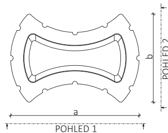
Pohled shora
