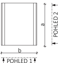
Pohled shora
