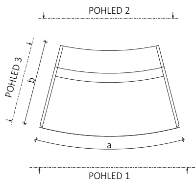
Pohled 1
