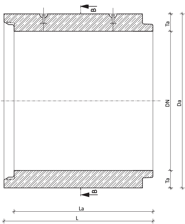
Řez A-A Trouba přímá (TBP / TZP)
