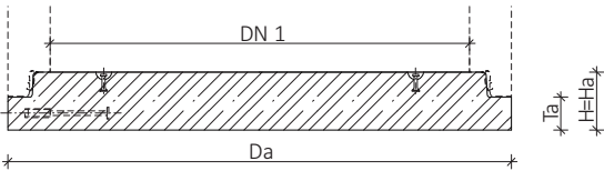
Deska pro dno šachty s IT pro DN 2000 až DN 3000
