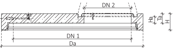
Deska přechodová s IT pro DN 2000 až DN 3000
