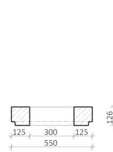
Řez B-B
