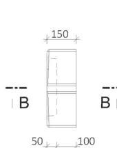
Pohled shora
