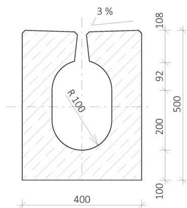
Řez A-A
