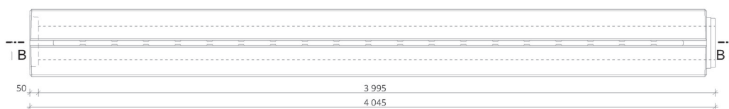
Pohled shora
