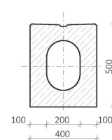
Řez C-C
