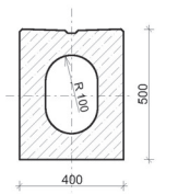
Řez C-C
