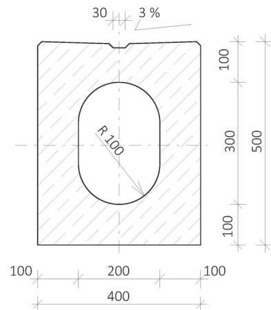
Řez C-C
