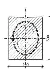
ŘEZ A-A
