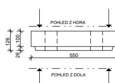
POHLED 2
