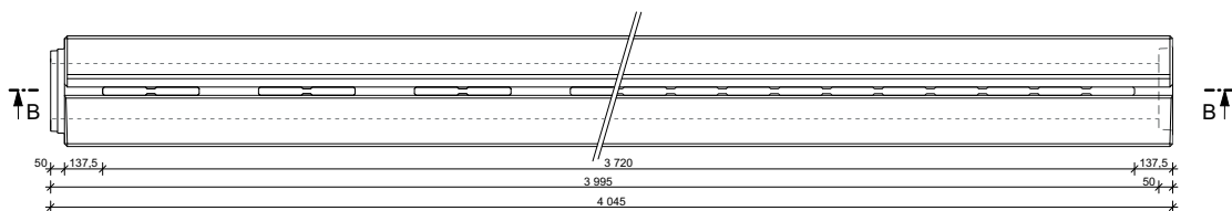
POHLED SHORA
