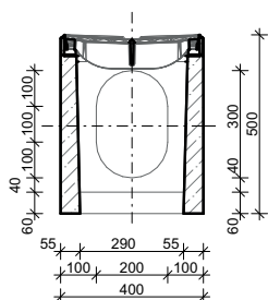
ŘEZ C-C
