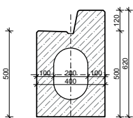
ŘEZ C-C
