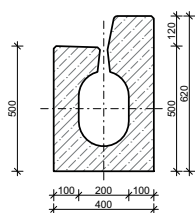
ŘEZ C-C
