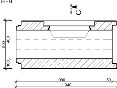
ŘEZ B-B
