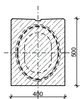
ŘEZ A-A
