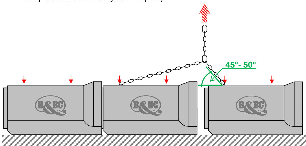
Obr. P1.3 Schéma sezazování trub řetězovým ukladačem.
