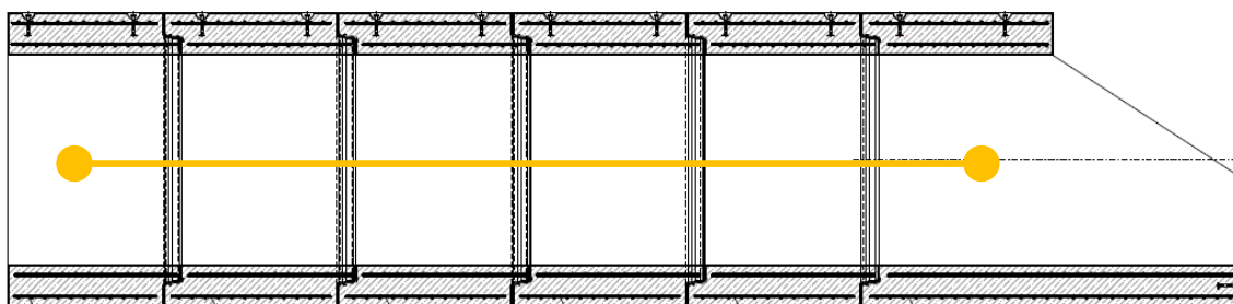
Obrázek P2.4 - Příklad celkové stažení celého propustku, na konci prací, je-li požadováno. Pro dodržení nedorazů (viz. článek 6.3) je vhodné dovnitř trub, do spojů, vsadit distanční vložky (např. dřevěné laťky).
